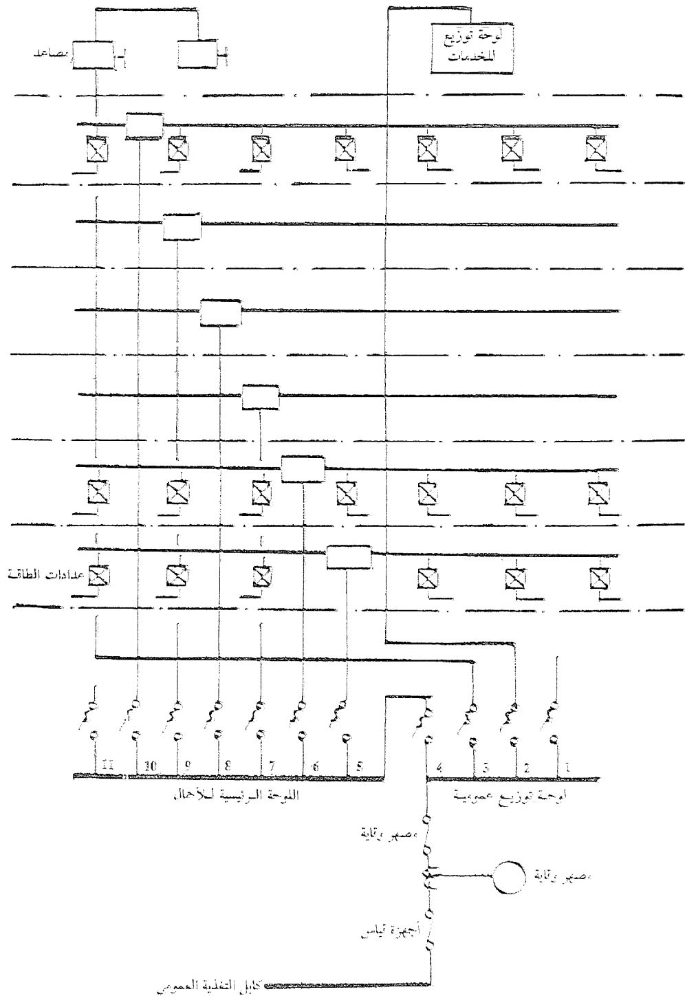
شكل رقم ( ٤ - ٢ ) نموذج التخطيط أحادي الخط لسار التيار
