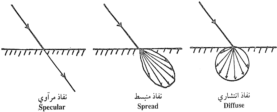
شكل رقم ( ٥ - ١٠ ) الأشكال المختلفة للنفاذ
